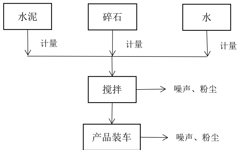
图 2-4 水稳料生产工艺流程图及产污环节
